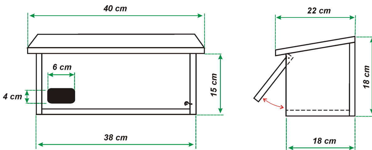
Rys. 2. Schemat budowy drewnianej skrzynki dla jерzyka
